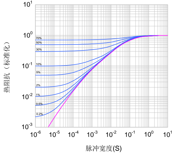
图 14. 瞬态热阻抗-脉冲宽度 (IGBT)
