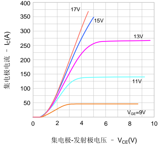
图2. 典型输出特性 (125°C)
