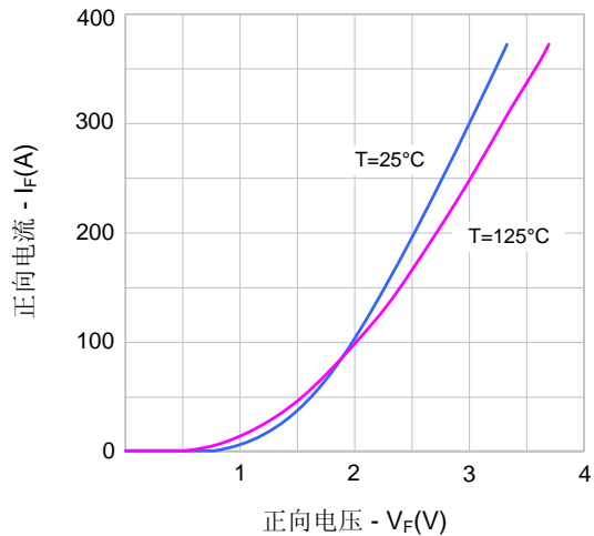
图 12. 二极管正向特性
