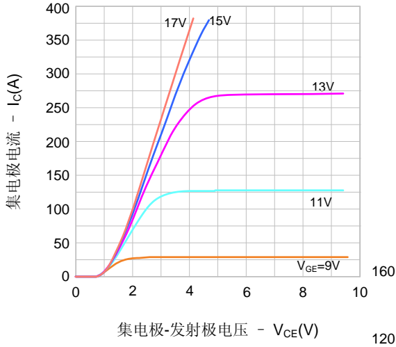
图1. 典型输出特性 (25°C)
