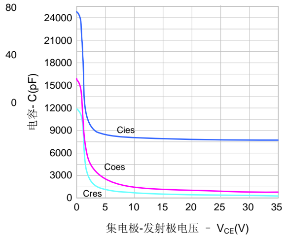
图4. 电容特性
