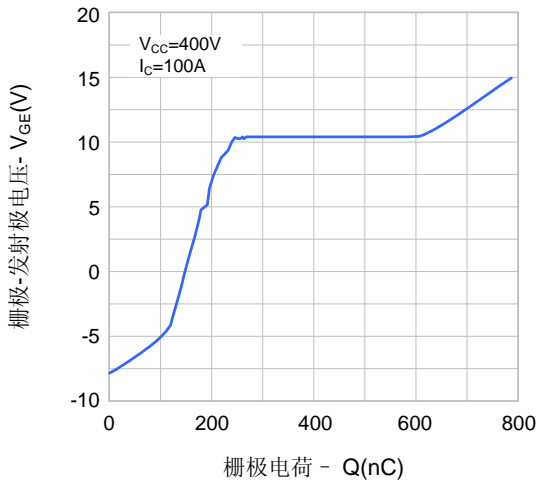
图 5. 栅极电荷特性
