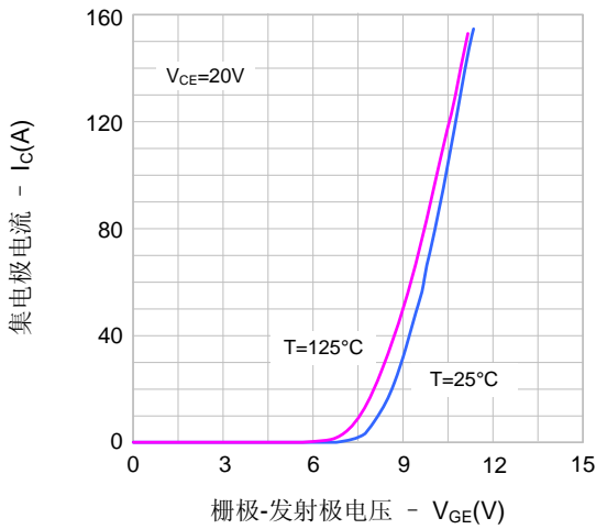
图3. 传输特性
