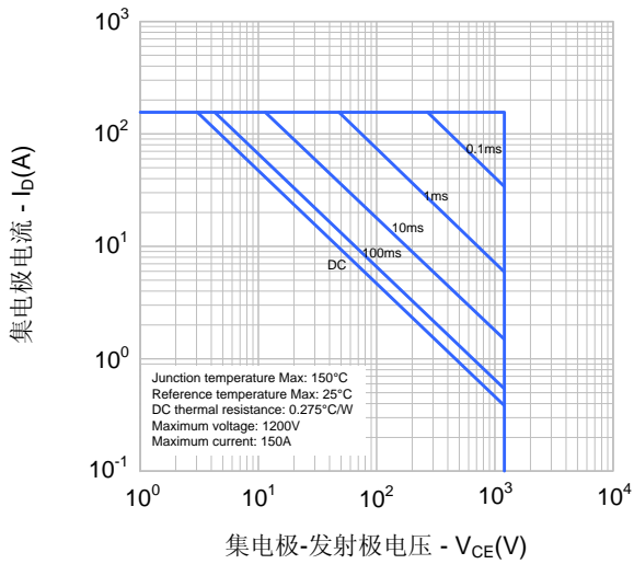
图15. 最大安全工作区域
