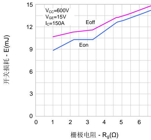
图8. 开关损耗 vs. 栅极电阻
