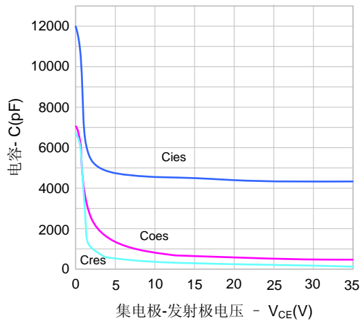
图4. 电容特性
