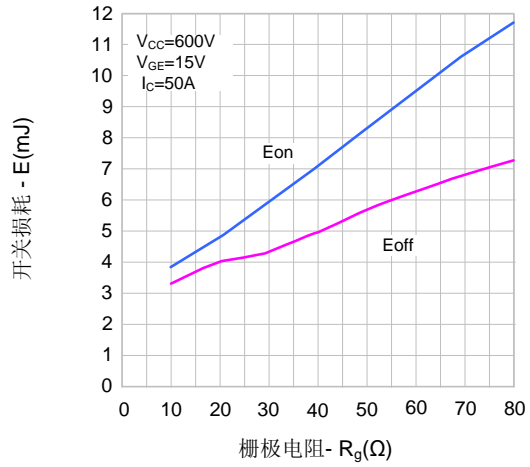
图8. 开关损耗 vs. 栅极电阻
