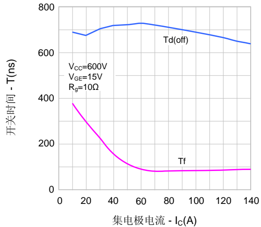
图10. 关断特性 vs. 集电极电流
