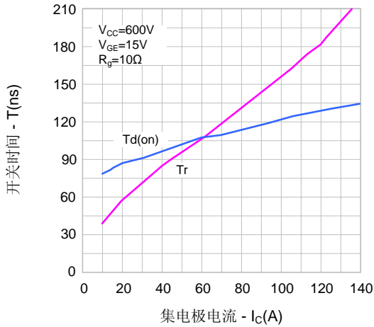
图9. 开启特性 vs. 集电极电流
