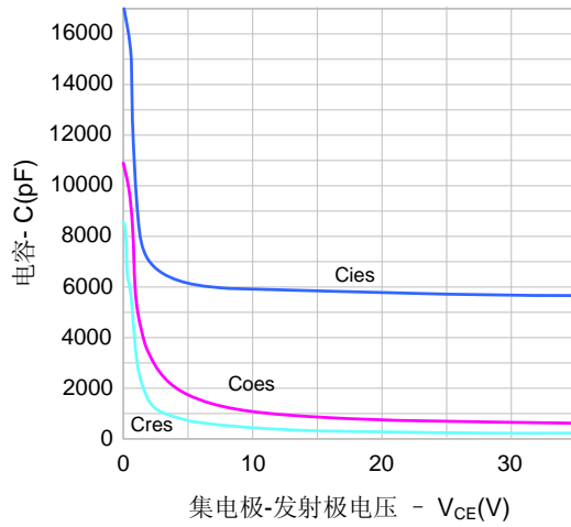
图4. 电容特性
