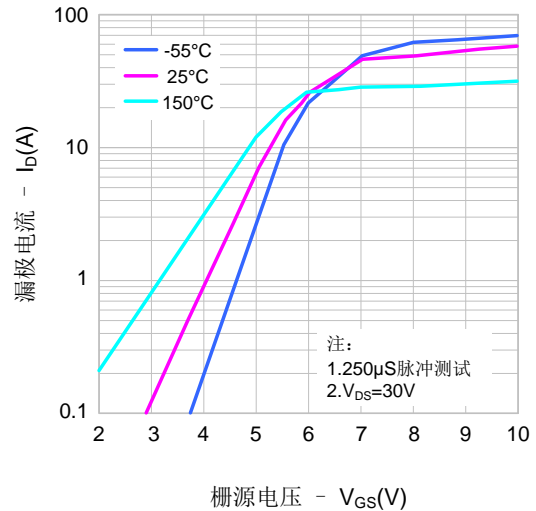
图2. 传输特性
