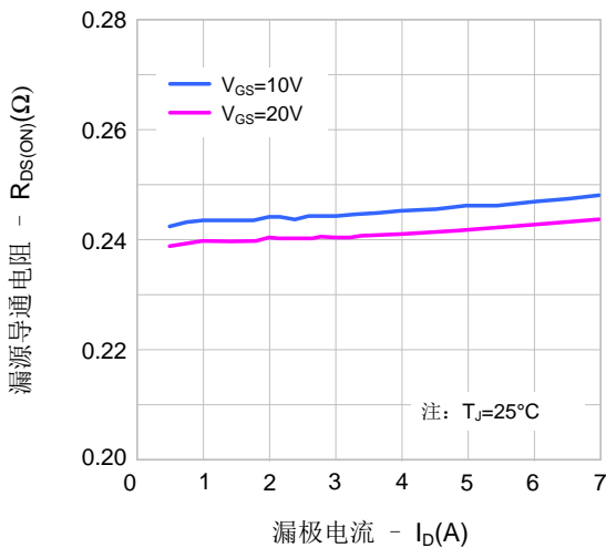
图3. 导通电阻 vs. 漏极电流、栅极电压
